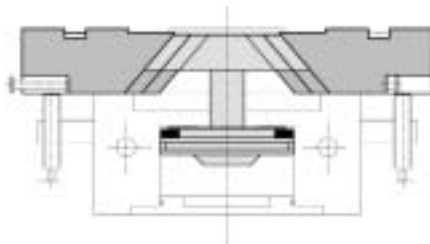
• SCHEMA DI FUNZIONAMENTO • OPERATIONAL DIAGRAM • BETRIEBSSCHEMA • SCHÉMA DE FONCTIONNEMENT
