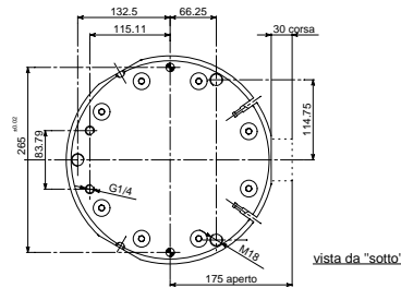
• Disegno QPG 330 • Drawing QPG 330 • Zeichnung QPG 330 • Dessin QPG 330
